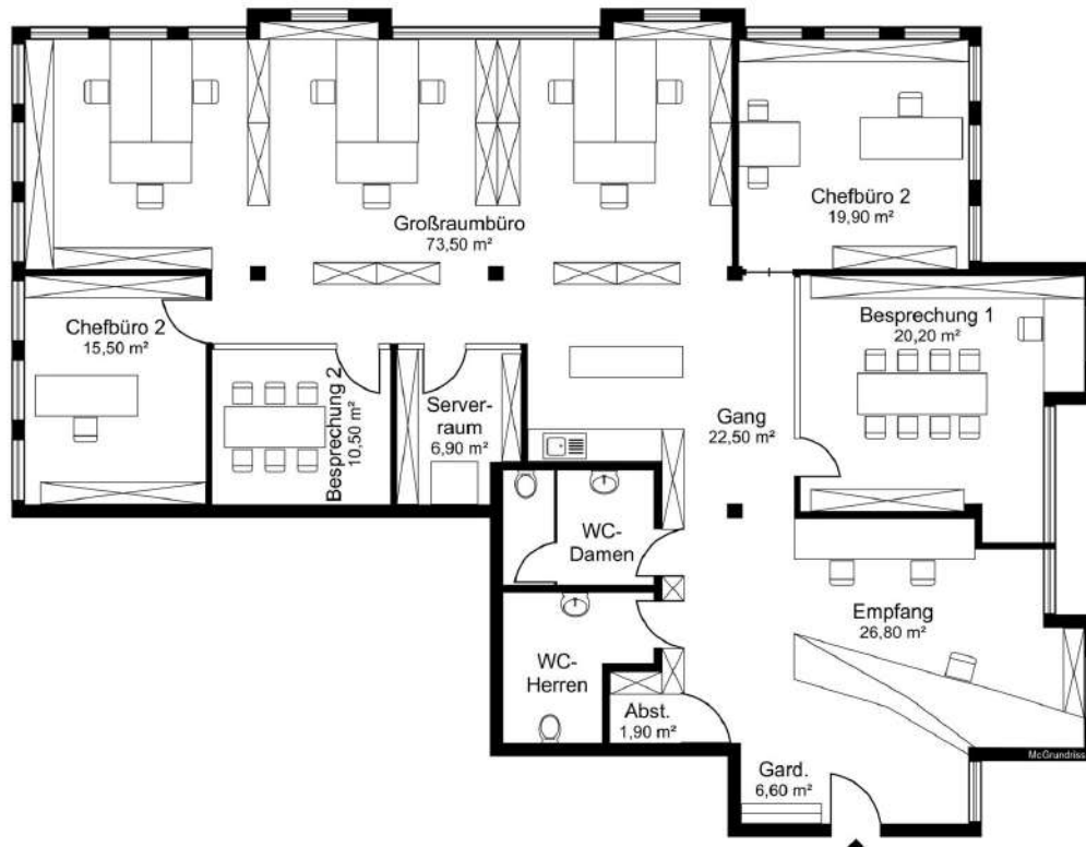
Grundriss
